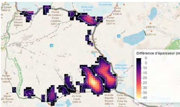
Perte d'épaisseur de glace
