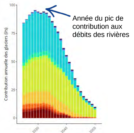
Contribution annuelle cumulée de la fonte de glace aux débits des rivières sur un bassin versant
